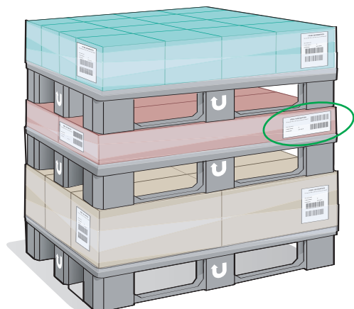
Placering av GS1 palletkett på lavpallar.
