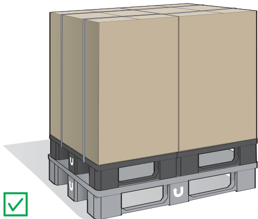
Exempel halvpall med wellpappshuv hur den ska förankras med plastband och placeras på slavpall.
