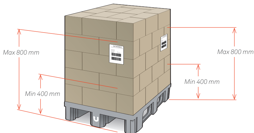
Etikettplacering av GS1 etikett på pallen.
